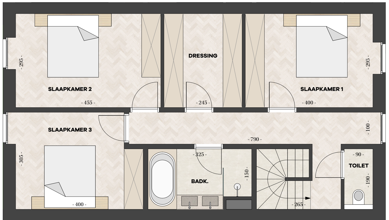
VERDIEPING +1
